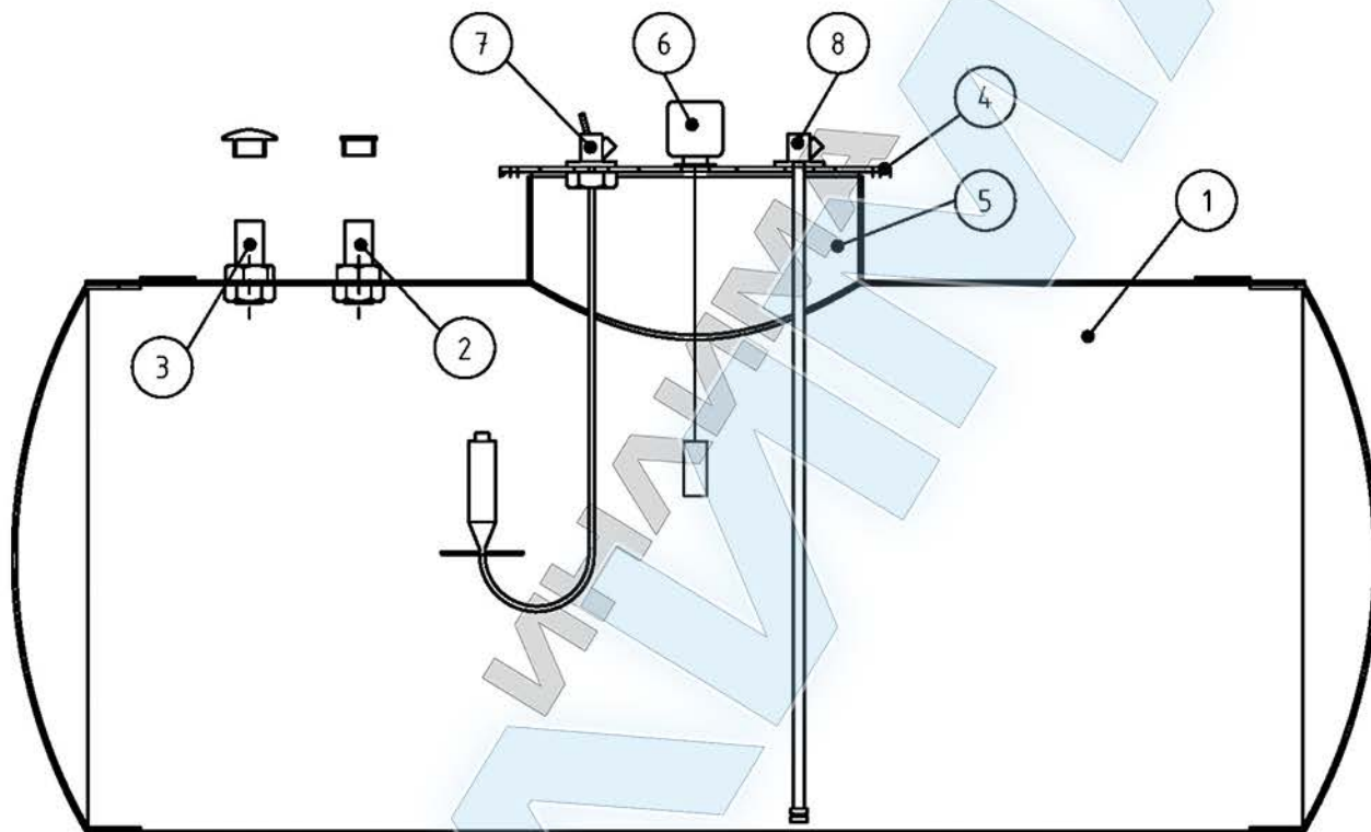
Рисунок 1. Общий вид (разрез) топливной емкости
